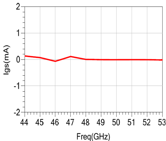
动态栅电流 vs. 频率@Pin=24dBm
