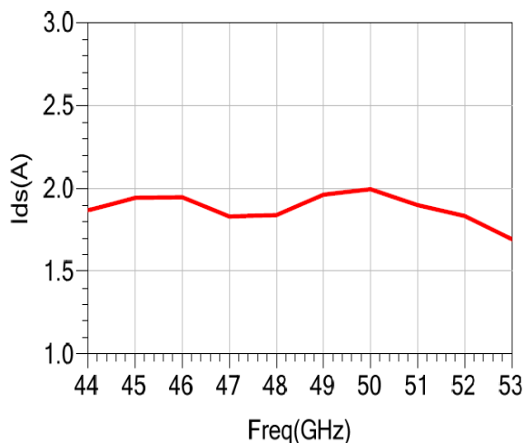
动态漏电流 vs. 频率@Pin=24dBm
