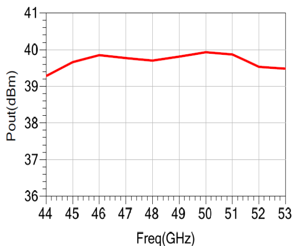
饱和输出功率 vs. 频率@Pin=24dBm
