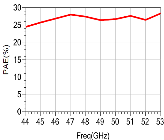
功率附加效率 vs. 频率@Pin=24dBm
